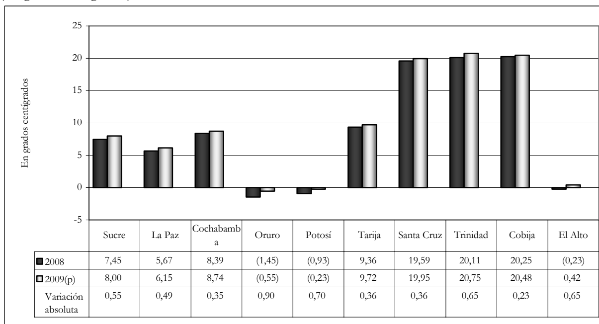
Gráfico N° 25 BOLIVIA: TEMPERATURA MÍNIMA AMBIENTE, SEGÚN CIUDAD CAPITAL, 2008-2009 (En grados centígrados)
