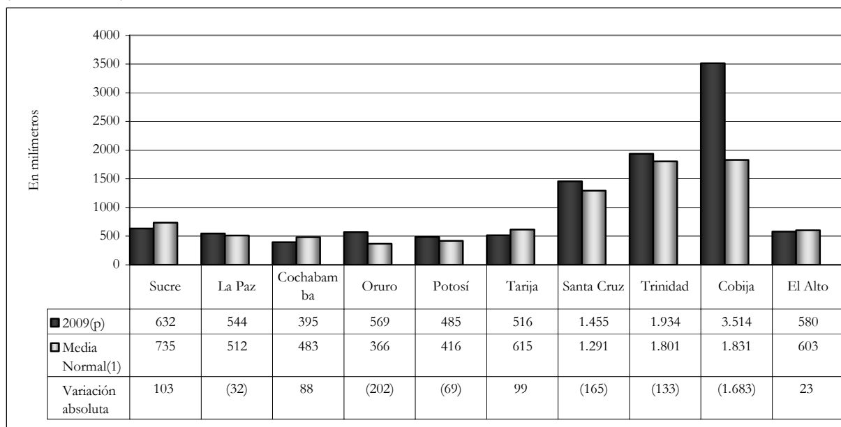
Gráfico N° 26 BOLIVIA: PRECIPITACIÓN PLUVIAL ACUMULADA, SEGÚN CIUDAD, 2009 (En milímetros)
